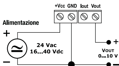
Fig.6: uscita analogica in tensione
