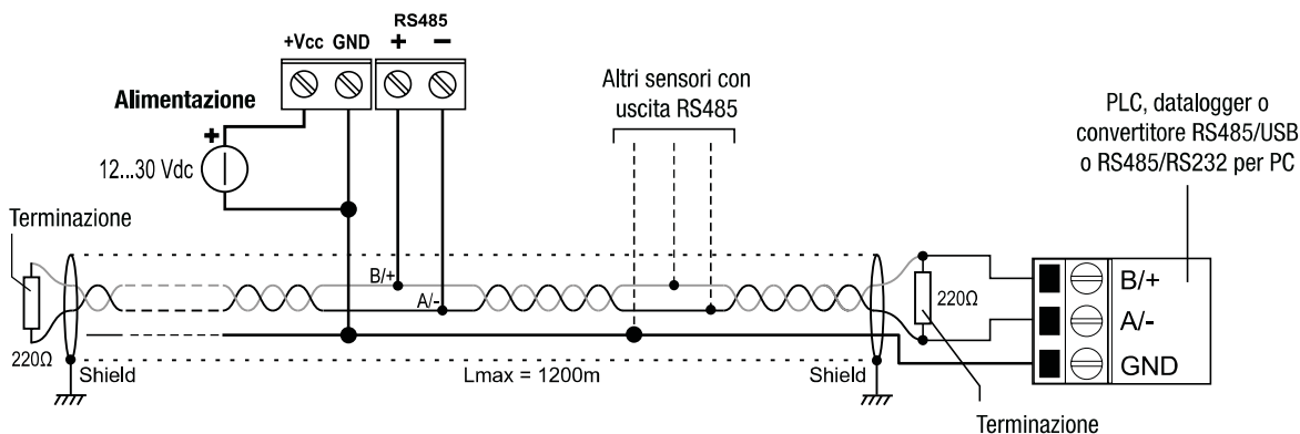
Fig. 7: Connessione RS485
