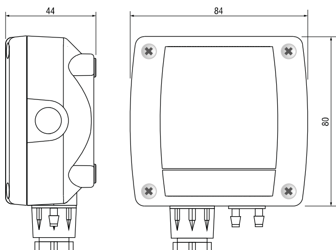
Fig. 2: dimensioni (mm)
