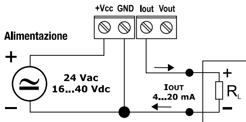
Fig. 4: uscita analogica in corrente
