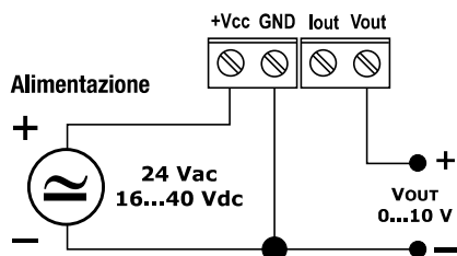
Fig. 5: uscita analogica in tensione
