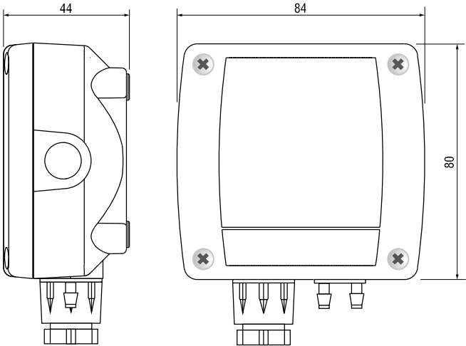
Fig. 1: dimensioni (mm)
