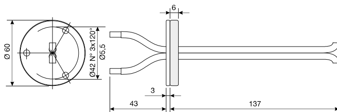
Fig. 7: sonda da canale AP3719
