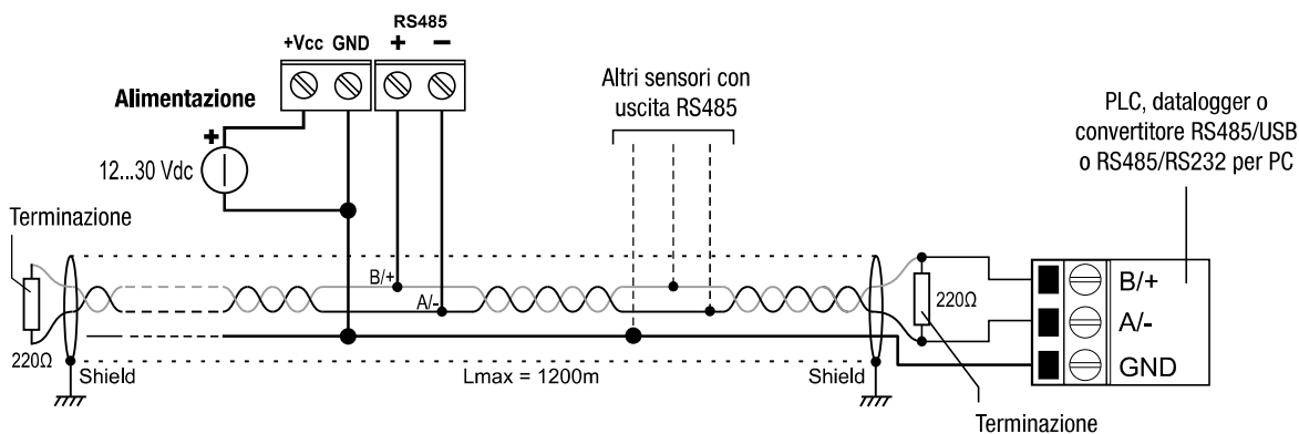
Fig. 6: Connessione RS485
