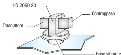
Fig. 5: Utilizzo di contrappesi
