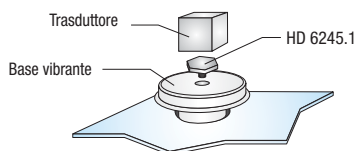
Fig. 3: Fissaggio del trasduttore mediante incollaggio
