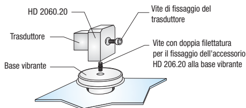
Fig. 4: Utilizzo dell'accessorio HD 2060.20
