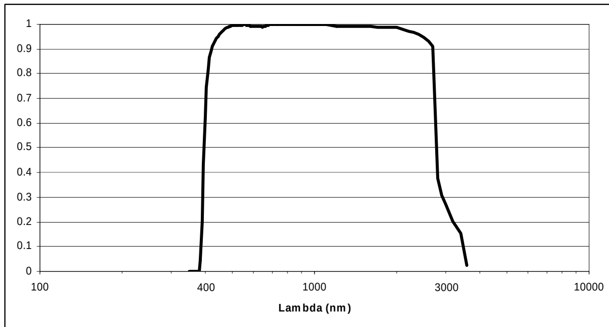
Figura 12: risposta spettrale del piranometro
