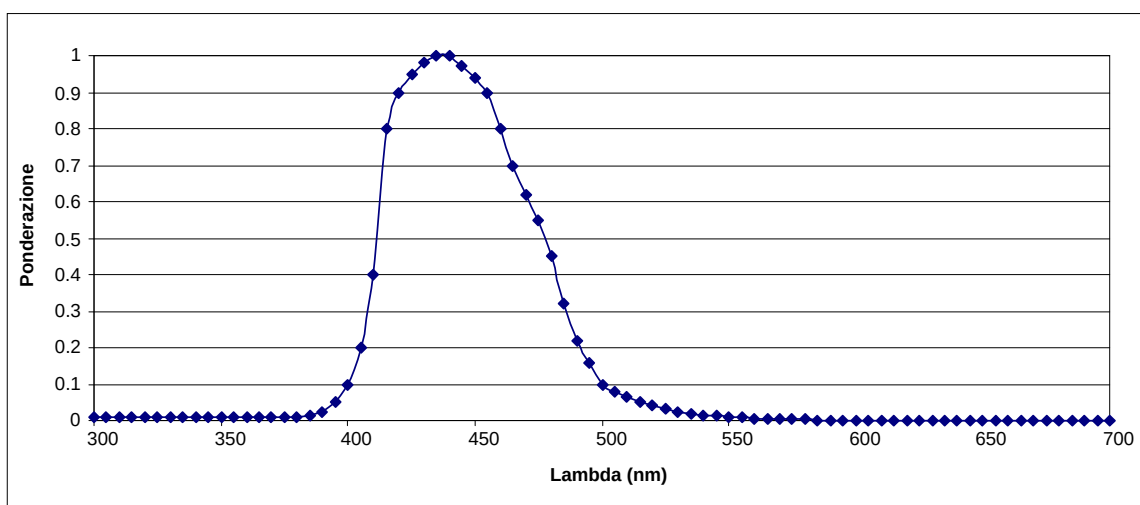
Figura 6: Curva di ponderazione spettrale B(\lambda)
