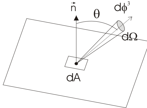
Figura 2: radianza
