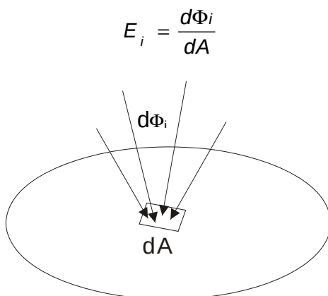
Figura 1: irradiamento
