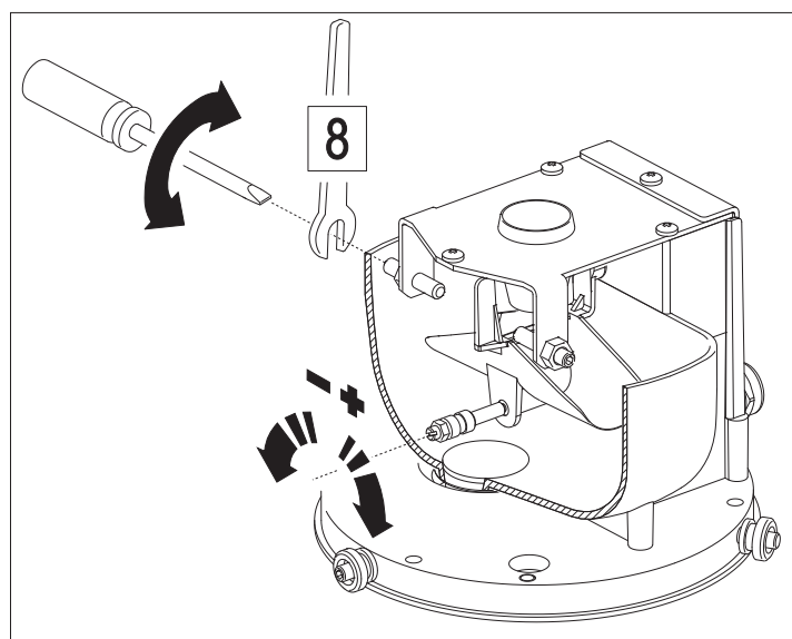
Fig. 4 - Regolazione della vaschetta basculante
