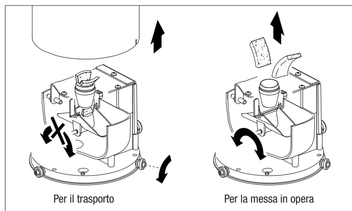
Fig. 3 - Bloccaggio e sbloccaggio della vaschetta basculante
