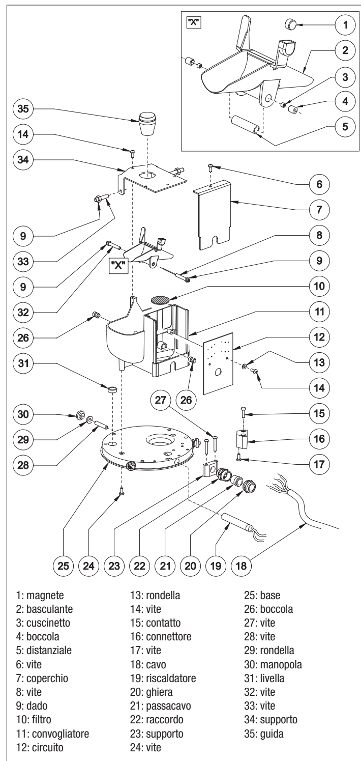
Fig. 9 - Esploso parte inferiore (versione con riscaldamento)
