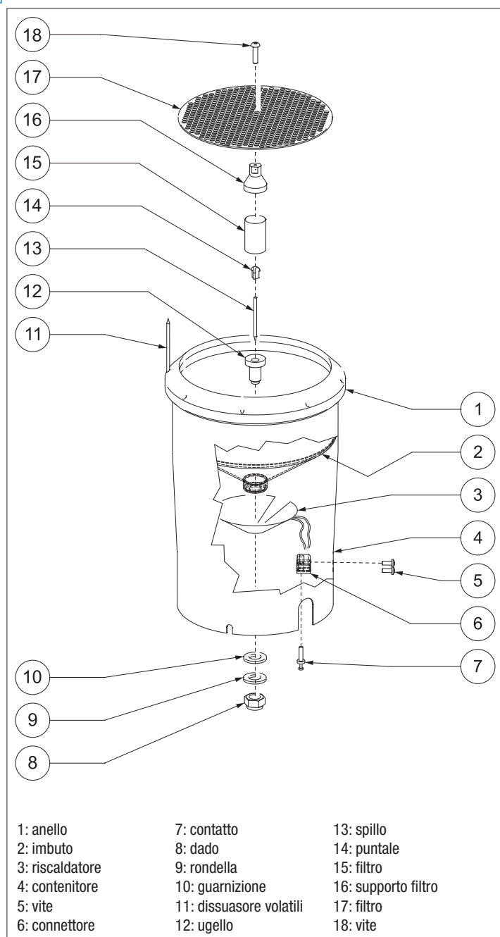
Fig. 10 - Esploso parte superiore (versione con riscaldamento)
