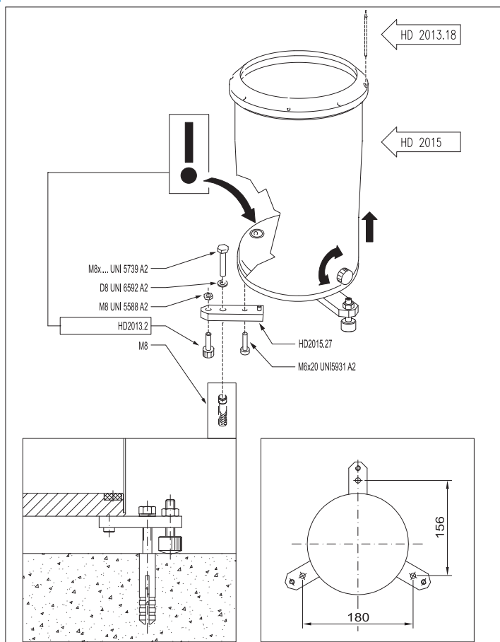
Fig. 7 - Installazione a pavimento
