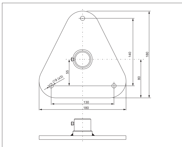
Fig. 6 - Base per fissaggio a pavimento (HD2013.78)
