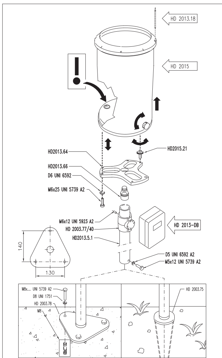
Fig. 8 - Installazione sollevato da terra
