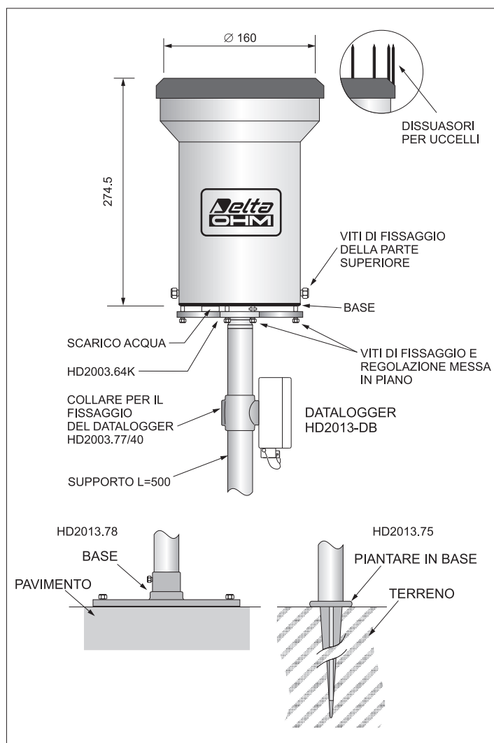
Fig. 5 - Dimensioni meccaniche, sistemi d'installazione
