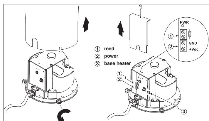
Fig. 2 - Connessioni elettriche (versione con riscaldamento)
